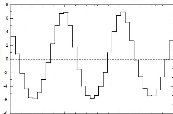
А. Изменение синодического периода Луны с течением времени (в часах). Среднее значение 29^{\text{d}} 12^{\text{h}} 44^{\text{m}}
